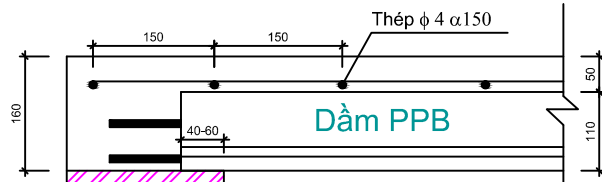
Chi tiết gối dầm PPB
