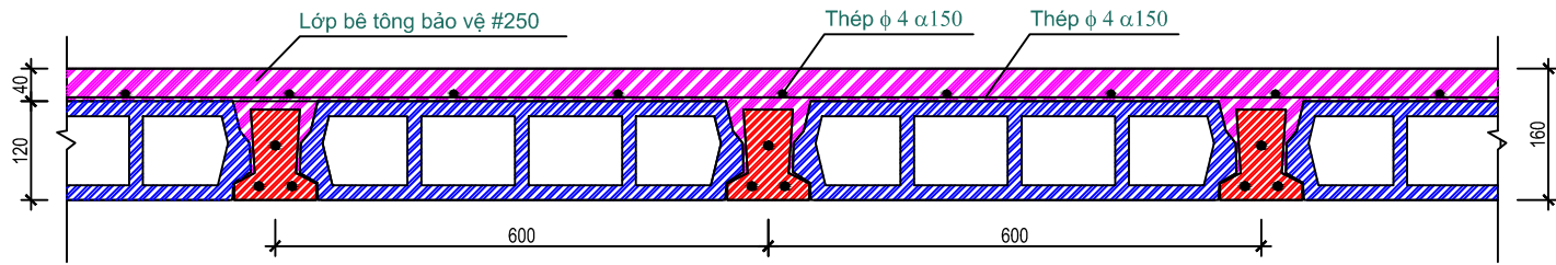
Mặt cắt chi tiết sàn PANEL nhẹ PPB
